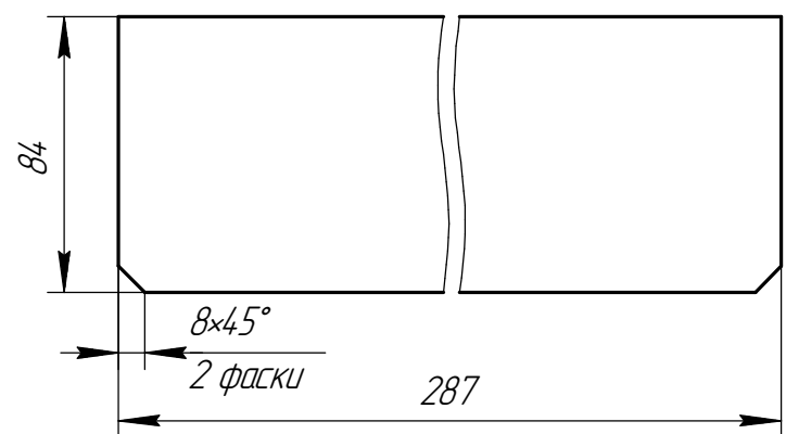
Дет. поз. 3 (1:2,5)
